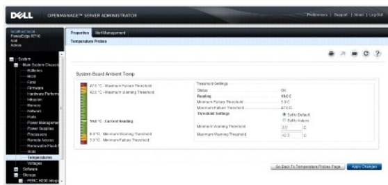
Abbildung 3-3. Messanzeige
